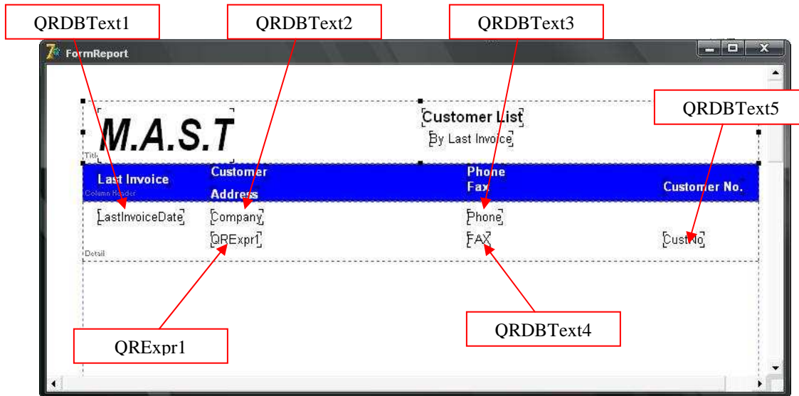
Gb. Penempatan QRDBText dan QRExpr pada DetailBand
